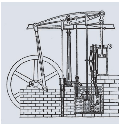
James Watt gőzgépe, amely képes volt az egyenes dugattyúrúd mozgását forgómozgássá átalakítani
